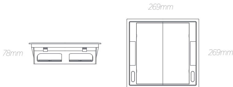
Teknik Çizim
