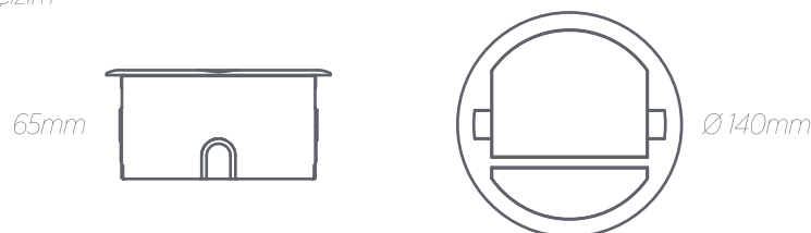
Teknik Çizim
